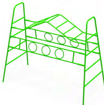
2248 Рукоход Размер: 2500 x 1300 x 2100
