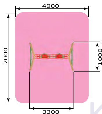
1115 Качели на столбах (двойные) Размер: 1000 x 3300 x 2000
