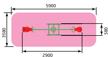
1480 Балансир металлический Размер: 2900 x 580 x 850
