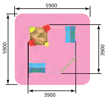
1233 Песочница "Морячок" Размер: 3900 x 3900 x 2500
