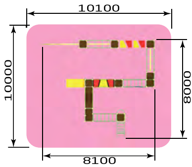
2209 Полоса препятствий 3 Размер: 8100 x 8000 x 2000
