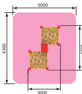
1203 Песочный дворик "Ракушка" Размер: 4300 x 3000 x 1850
