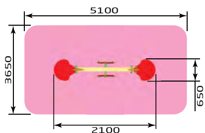
1407 Балансир "Забава" (одинарная) Размер: 2100 x 650 x 700
