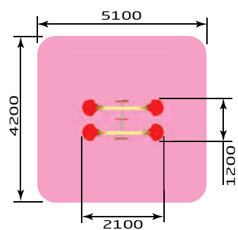
1408 Балансир "Забава" (двойная) Размер: 2100 x 1200 x 700
