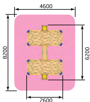
1202 Песочный дворик "Орешек 2" Размер: 6200 x 2600 x 1600
