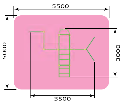
2102 Спорт комплекс "Минимакс" Размер: 3000 x 3500 x 2300
